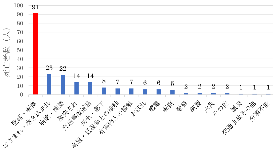
建設業における事故の型別死亡災害発生状況（令和7年）
